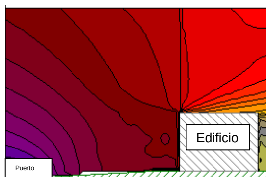
L den : Sección sobre Predicción sonora Puerto-Edificio más próximo
