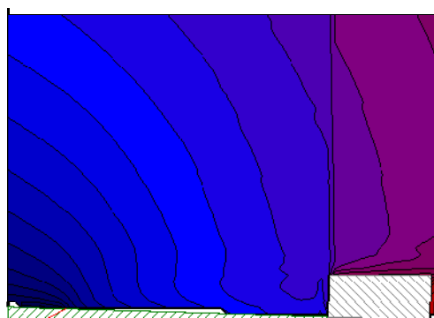
L den : Sección sobre Predicción sonora Fábrica Cemento-Edificio más próximo
