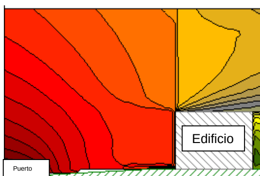
L night : Sección sobre Predicción sonora Puerto-Edificio más próximo
