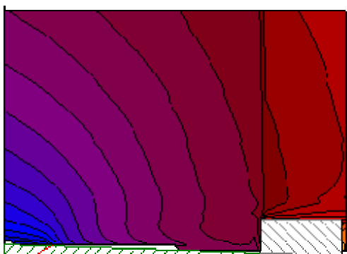
L night : Sección sobre Predicción sonora Fábrica Cemento-Edificio más próximo
